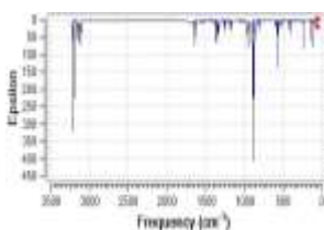
Coronene-Zn
