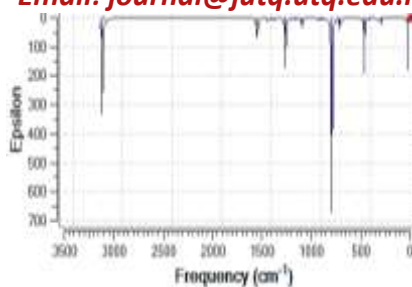
Coronene
