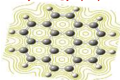
Coronene
