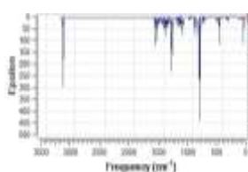
Coronene-S
