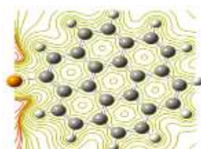
Coronene-P
