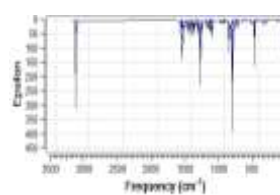
Coronene-Se
