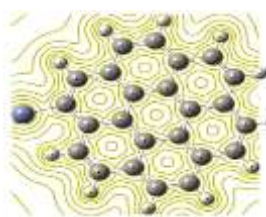
Coronene-Zn
