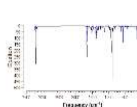
Coronene-F
