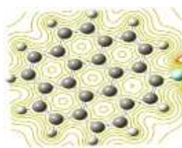
Coronene-F
