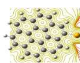
Coronene-S
