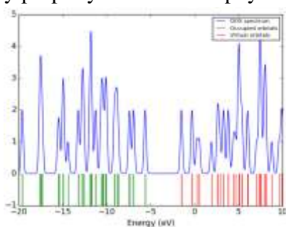
Coronene
